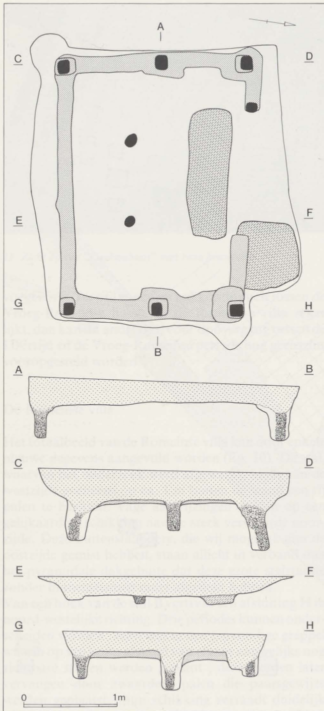
13 Plattegrond en doorsneden van een "weefhut".
