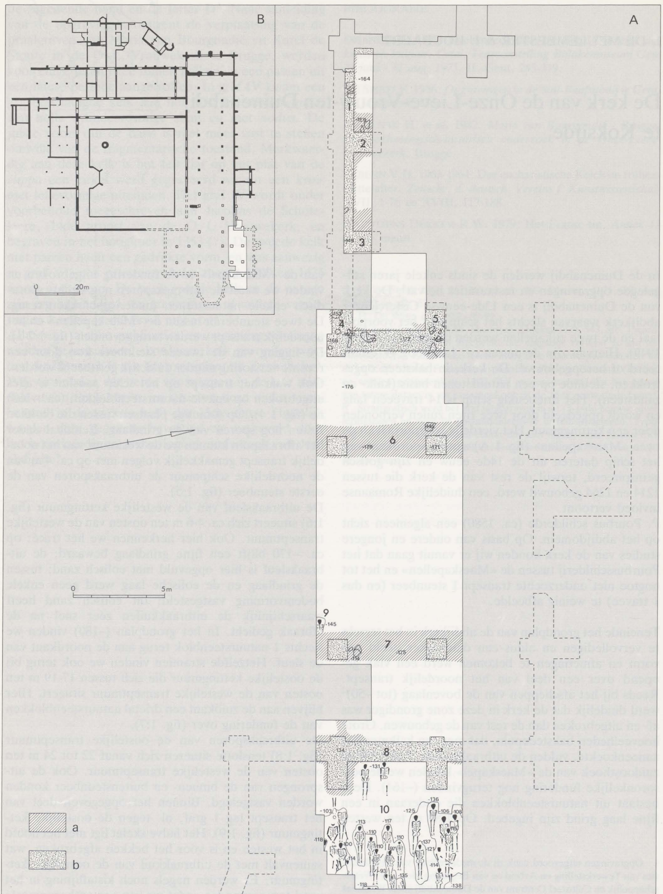
1 Vereenvoudigd opgravings- en interpretatieplan (A) met situering van het plan binnen de ruïnes (B): a. uitbraaksleuven; b. restitutie van de kerkmuren binnen de uitbraaksleuven (verdere legende verklaard in de tekst).
