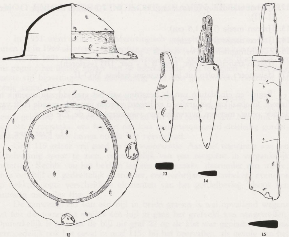
Fig. 53. — Wapens uit het Merovingische grafveld op de Eindhovenakker (12-15: sch. 1/3).
