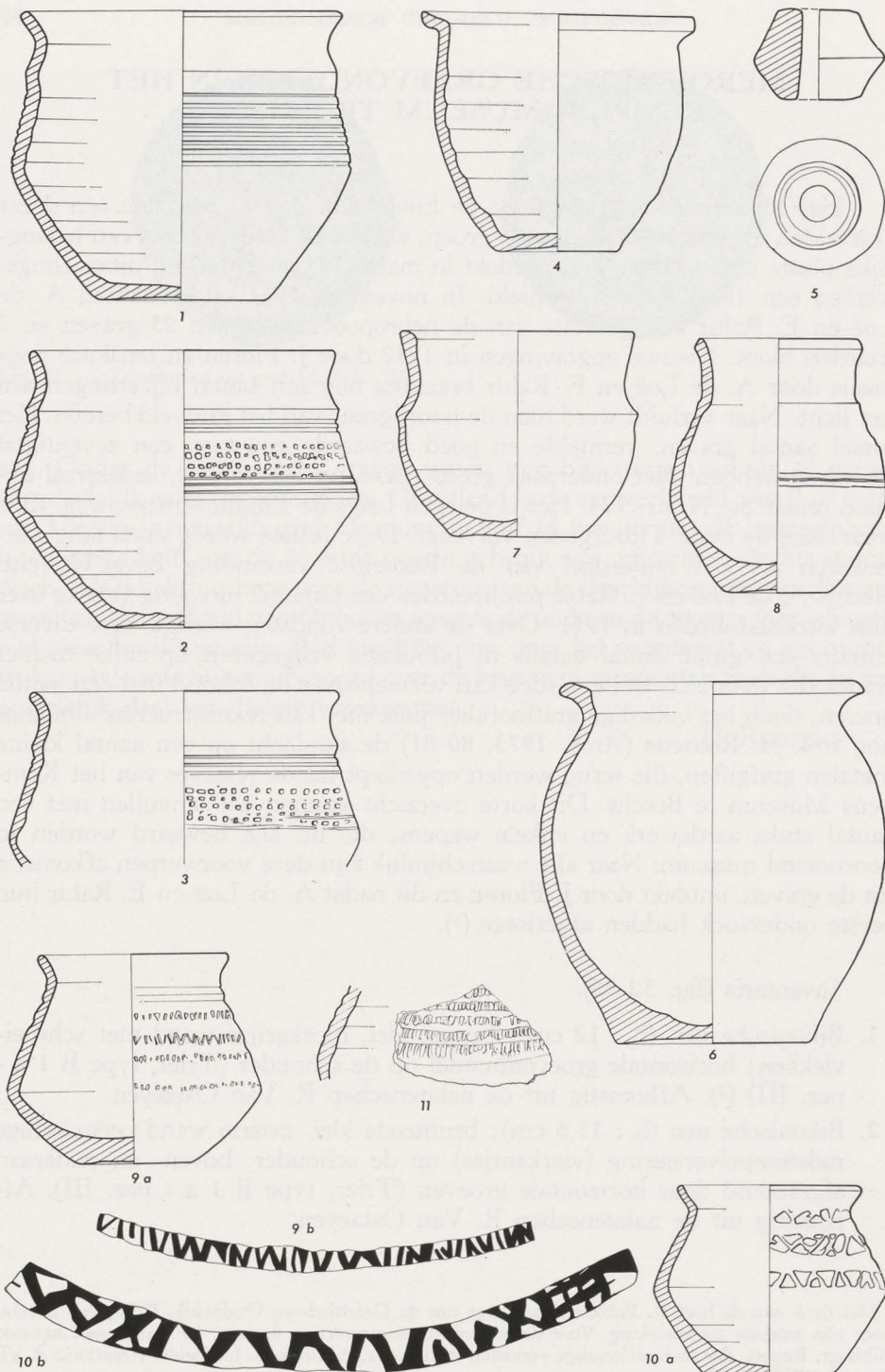
Fig. 52. — Aardewerk uit het Merovingisch grafveld op de Eindhovenakker (sch. 1/3; 9 b en 10 b: sch. 2/3).
