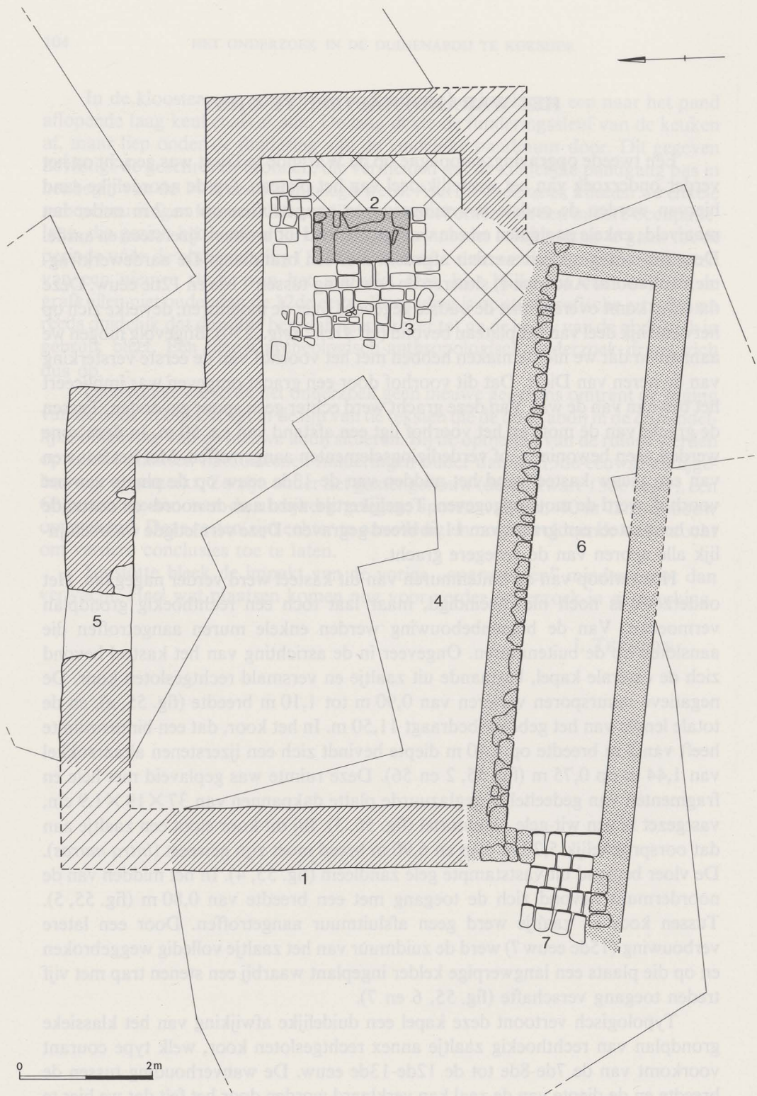
Fig. 55. Algemeen plan van de castrale kapel en de later toegevoegde kelder.
