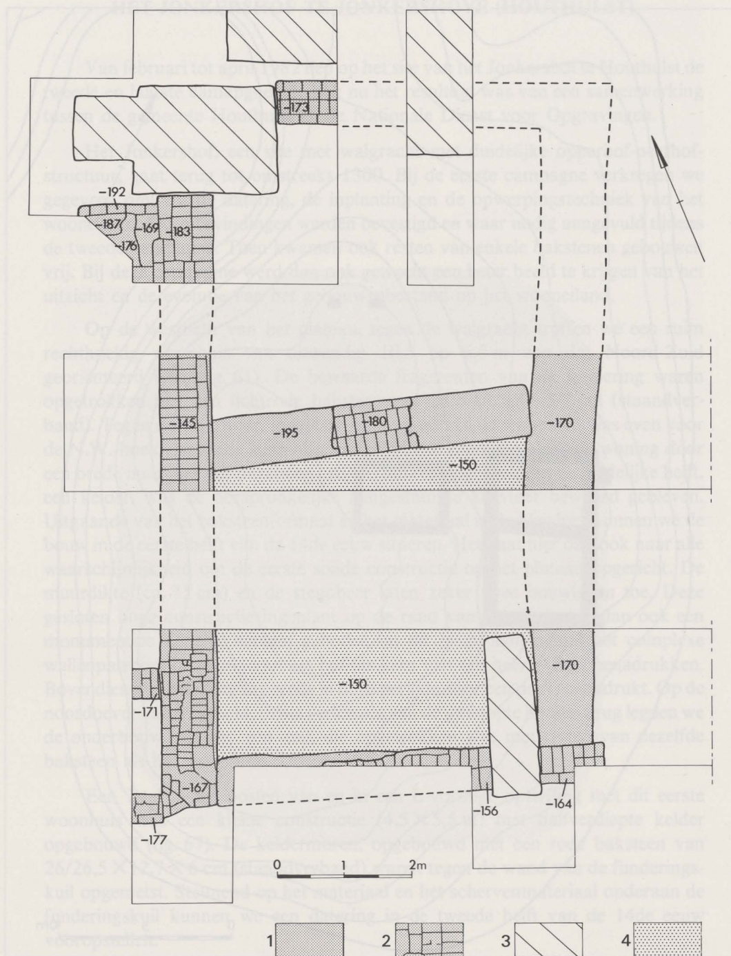
Fig. 62. Grondplan van het 14de-eeuwse woonhuis. 1 : uitbraak, 2 : in situ bewaarde funderingen, 3 : post-middeleeuwse constructies, 4 : keldervloer.
