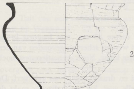
(Schaal 1: 6)
