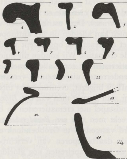
Afb. 20 (Schaal 1:3)
