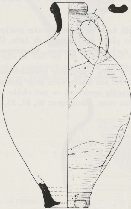
Afb. 16 (Schaal 1:3)
