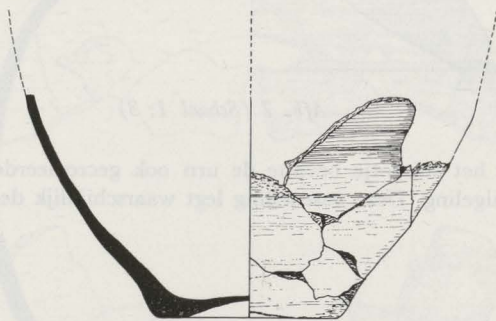
Afb. 6 (Schaal 1: 3)
