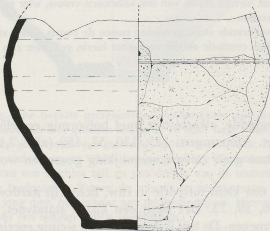
Afb. 8 (Schaal 1: 3)
