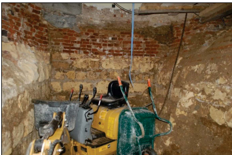
FIG.48 Zicht op de noordelijke en westelijke fundering van de kelder.
