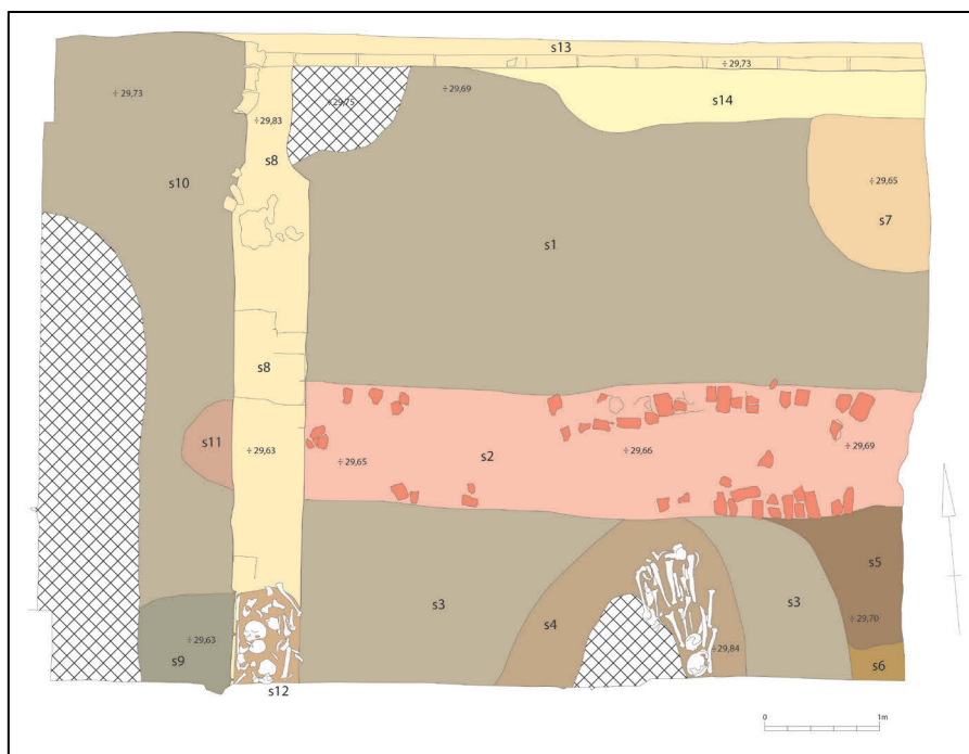
FIG. 19 Overzichtsplattegrond van de aanwezige sporen in werkput 1, vlak 1.
