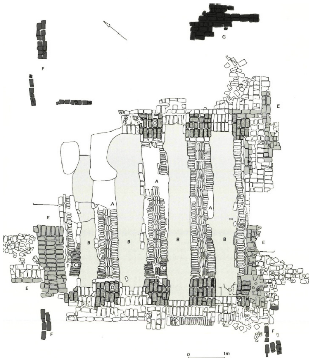
Figuur 38: Plattegrond van de goed bewaarde veldoven in de Achterhaven van Zeebrugge met interpretatie van de aangetroffen sporen: A. Stapelrijen; B. stookgangen; C. roze, misbaksels; D. muurdammen; E stenen die buitenste stapelrijen begrenzen; F: deel van muur rond veldoven; G: oudere fase van de oven (bron: Patrouille 2002, 248, fig. 6).
