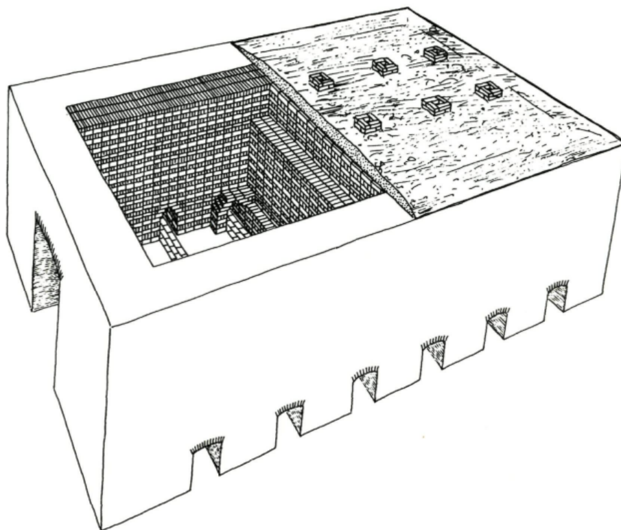
Figuur 43: Reconstructietekening van een laat-middeleeuwse baksteenoven. In: Devliegheer 1979, 280.
