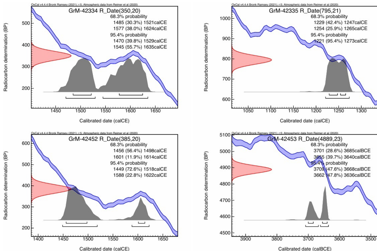
Figuur 35: Kalibratiecurves voor ^{14}\text{C} (M-1: GrM-42334; M-2: GrM-42335; M-3: GrM-42452; M-4: GrM-42453) (Kamjan 2026).
