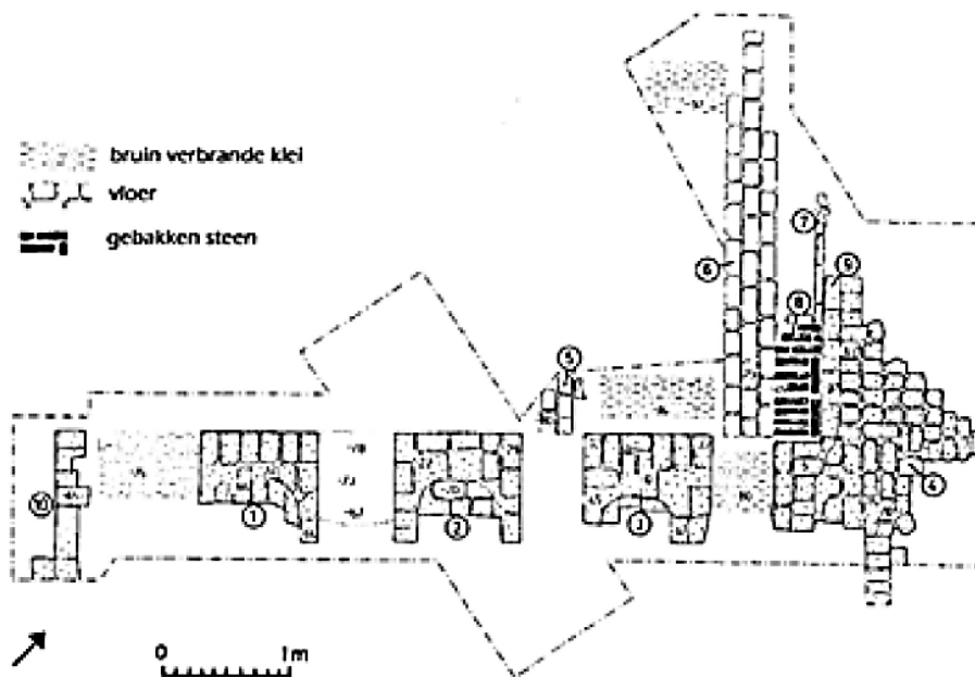
Figuur 37: Plattegrond van de fragmentair bewaarde veldovens op het domein Ayshove (Ramskapelle bij Zeebrugge) met interpretatie van de aangetroffen sporen (foto opgehaald uit: Devliegheer, 1979, 276).
