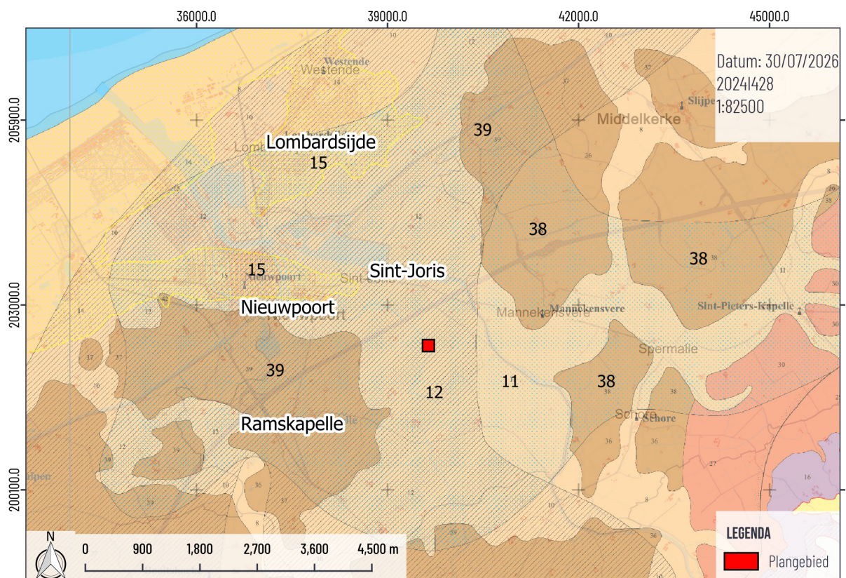
Figuur 10: Quartairgeologische profieltypekaart 1/50.000 met aanduiding van het plangebied en de relevante omliggende profieltypes. Bron: www.dovvlaanderen.be (8 juni 2026).
