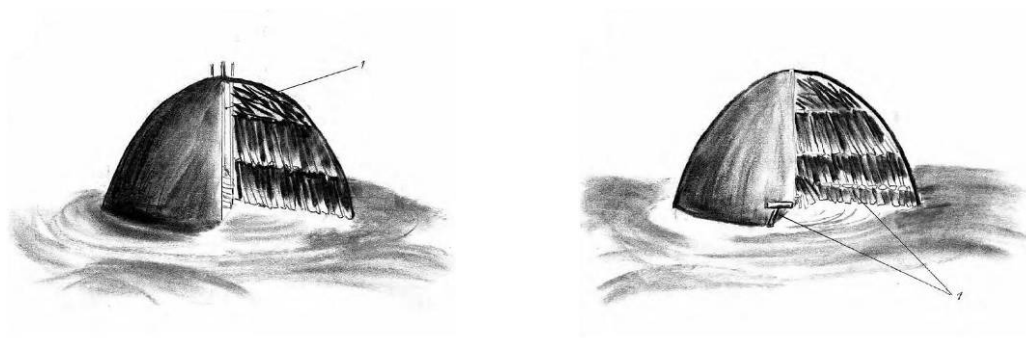
Fig. 3.1 Platzmeiler die aangestoken kan worden langs boven (links), waarbij 4 palen die boven aan de meiler uitsteken het onstekingskanaal markeren waarlangs de meiler met gloeiende houtskool in brand wordt gezet, of langs onder (rechts), waarbij de meiler door een onstekingskanaal (1) onderaan met behulp van een staaf in brand wordt gezet.
