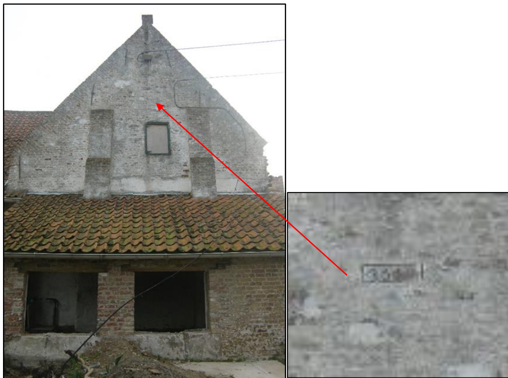
Fig. 5 Westgevel van het Spycgergoed, waarop de bouwdatum (1556 is aangebracht. Met steunberen en aandak.
