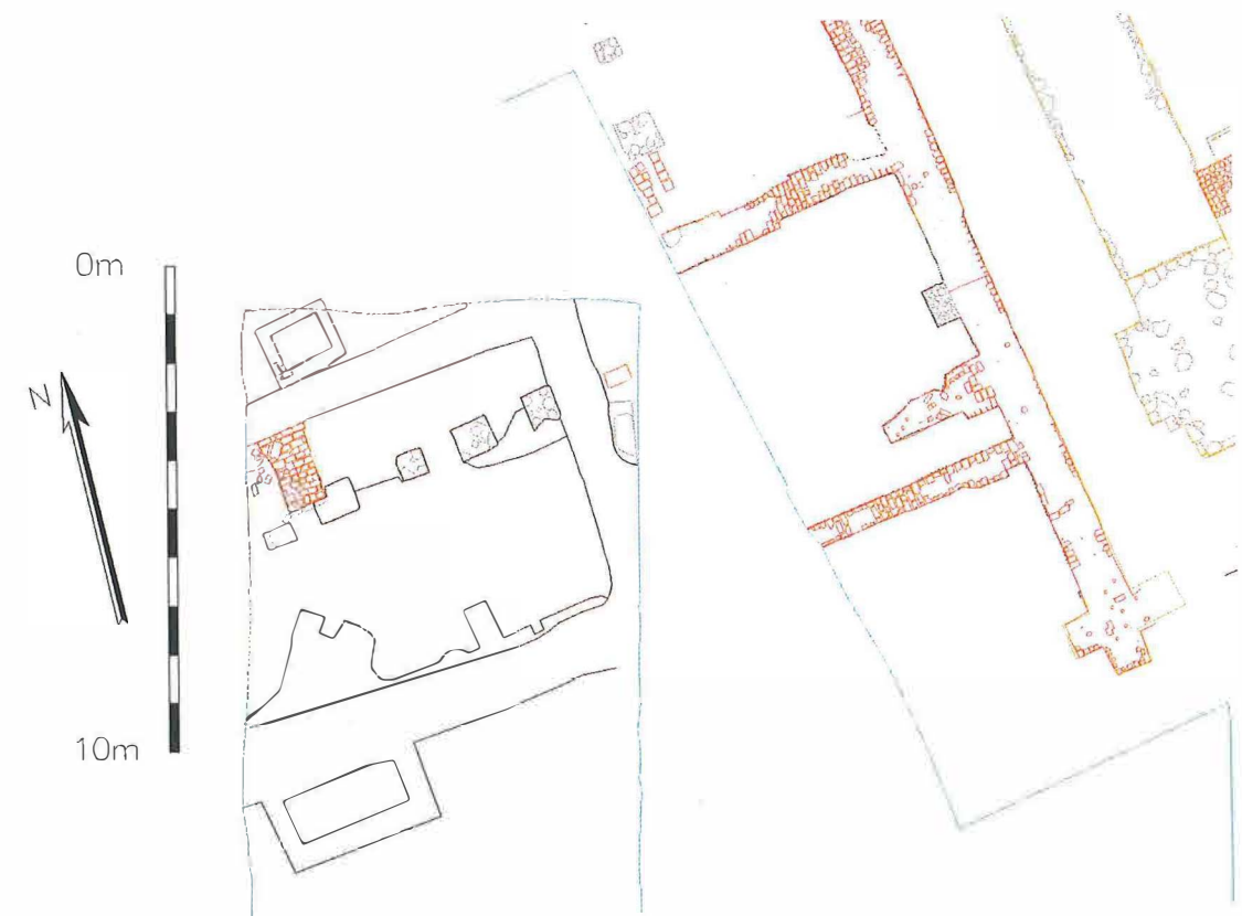
Figuur 4.8: Opgravingsplan van het gastenverblijf.
